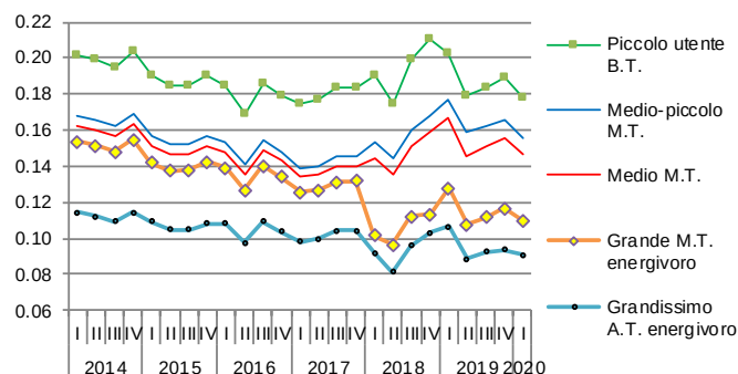
Figura 6.41 – Prezzi totali per diverse tipologie di imprese, incluse accise ed esclusa IVA (€/kWh).
