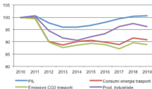
Figura 5.7 - Emissioni di CO 2 e consumi di energia del settore trasporti, PIL e produzione industriale (2010=100)
