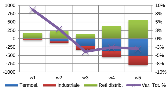
Figura 1.10 – Consumi di gas naturale per usi termoelettrici nel mese di marzo (var. tendenziale in Mni SMC su asse sin e % su asse dx) e domanda el. (var.% asse dx)
