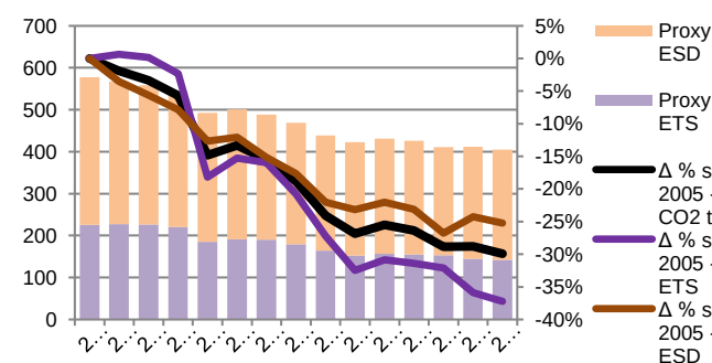
Figura 5.1 – Emissioni del sistema energetico italiano per settore (Mt CO 2 eq) e variazione % rispetto al 2005 (asse dx)
