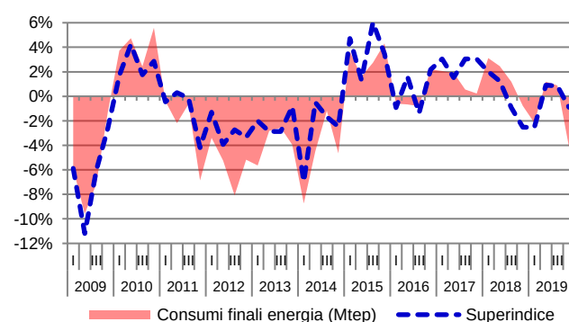
Figura 4.2 – Consumi finali di energia e Superindice ENEA (variazione su anno precedente, %)
